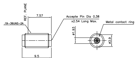
Bulkhead Receptacle Jack
